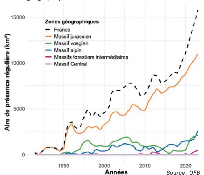
Evolution de l'aire de présence régulière du lynx par zone géographique de 1983 à 2023
