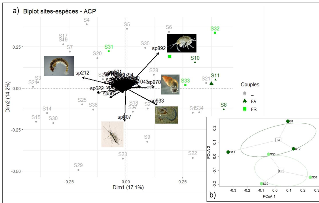
Figure 6 : a) Analyse en Composantes Principales (ACP) des abondances (préalablement Hellinger-transformées) de macroinvertébrés sur l'ensemble des 36 stations. Une minorité d'espèces très abondantes va a priori influencer la différenciation des sites, notamment les Chironomidae (sp807), Hydropsyche (sp212), gammarus (sp892), hydrobies (sp978) et oligochètes (sp933). b) Exploration graphique des assemblages en stations-cibles FA et FR via une Analyse en Coordonnées Principales (ACoP) sur la base des distances inter-sites de Bray-Curtis.
