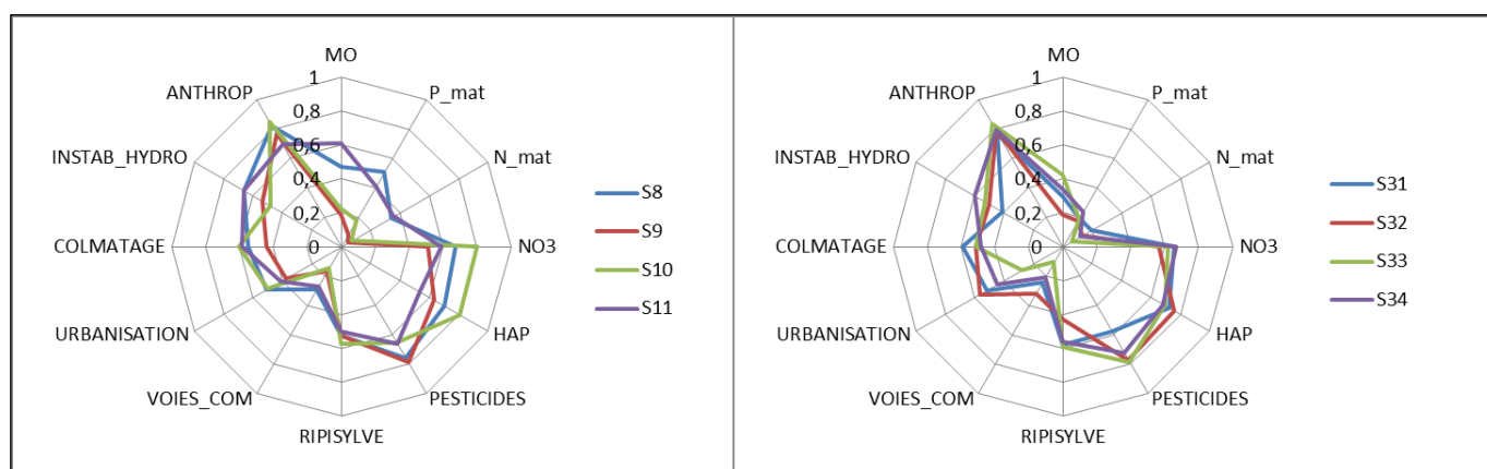
Figure 4 : Diagramme radar des probabilités de pressions sur les stations à RA (partie gauche) et à RR (partie droite).
