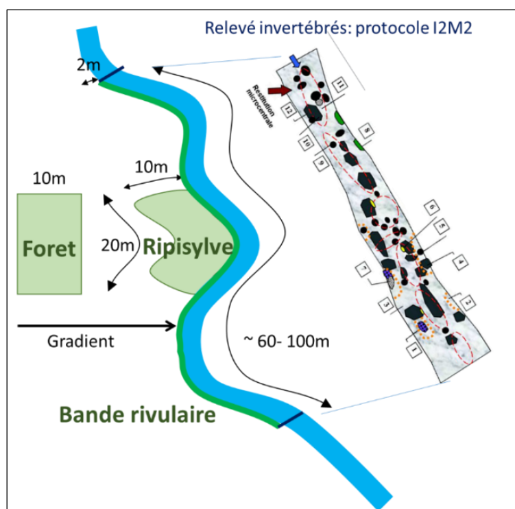
Figure 2 : Schématisation du protocole d'échantillonnage des divers compartiments : forêt, ripisylve, bande rivulaire et cours d'eau.
