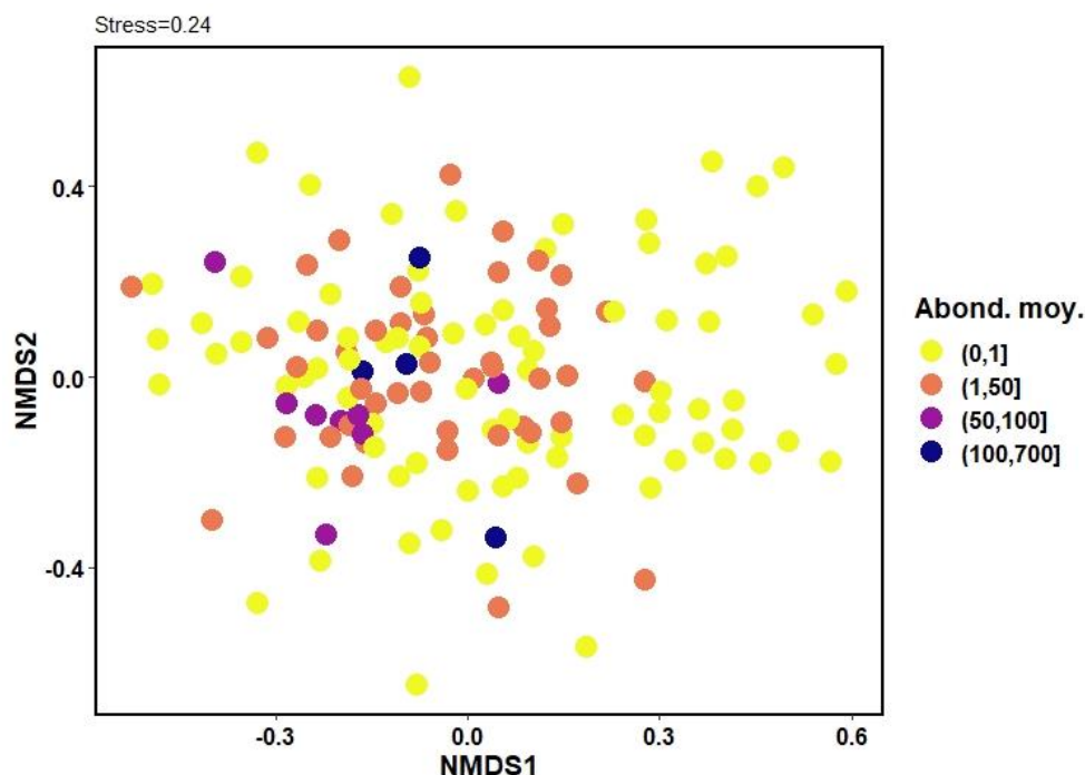
Figure 8 : Résultats de l'Analyse d'ordination Multidimensionnelle Non-Métrique (Non-Metric Multi-Dimensional Scaling) des taxons de macroinvertébrés (points) dans l'espace des 118 modalités de traits fonctionnels que nous avons réduit à deux dimensions (NMDS1 et NMDS2, R^2=0.73 , stress=0.24). La couleur des points indique la classe d'abondance moyenne des taxons.
