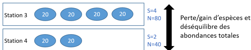
Figure 7 : Adapté de Baselga (2013). Schéma représentant les deux principaux processus sous-tendant potentiellement la diversité de composition taxonomique entre les stations (diversité beta) dans notre zone d'étude. Les valeurs sont uniquement à titre d'exemple. S=nombre d'espèces, N=abondances totales par site.
