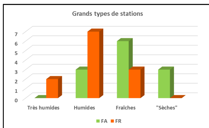
Figure 2 : Nombre de placettes de forêt ancienne (FA) et de forêt récente (FR) suivant les grands types de stations.
