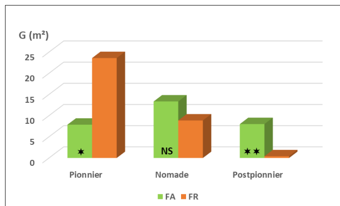
Figure 3 : Répartition de la surface terrière (G en m²/ha) suivant l'affectation des espèces d'arbres aux 3 stades de la succession dendrologique et suivant l'ancienneté de la forêt.
