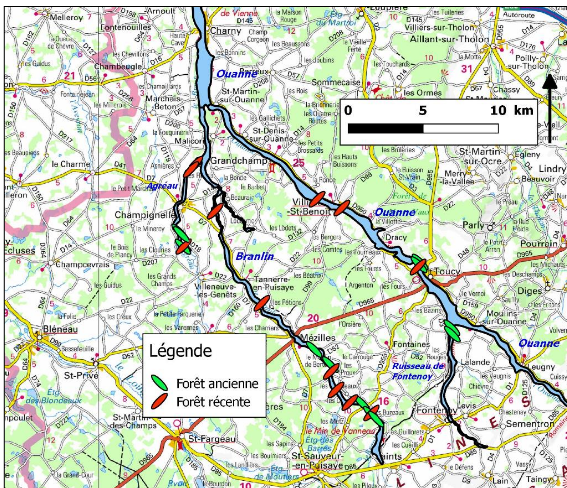
Figure 1 : Emplacement des points d'échantillonnage des forêts anciennes et récentes. (Fond de carte : IGN 1/250 000 ème ).
