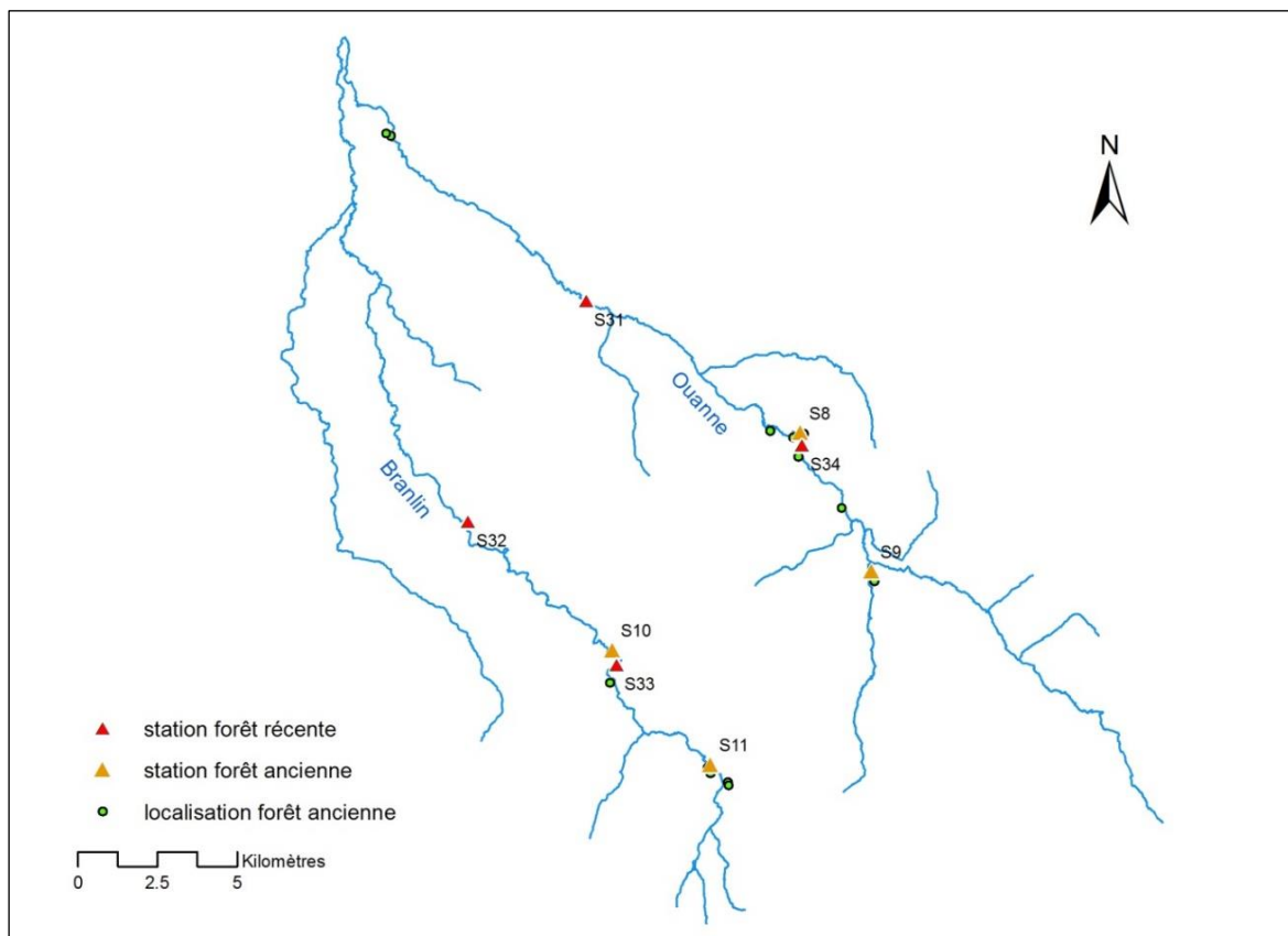
Figure 1 : Localisation des huit stations d'échantillonnage des macroinvertébrés benthiques.
