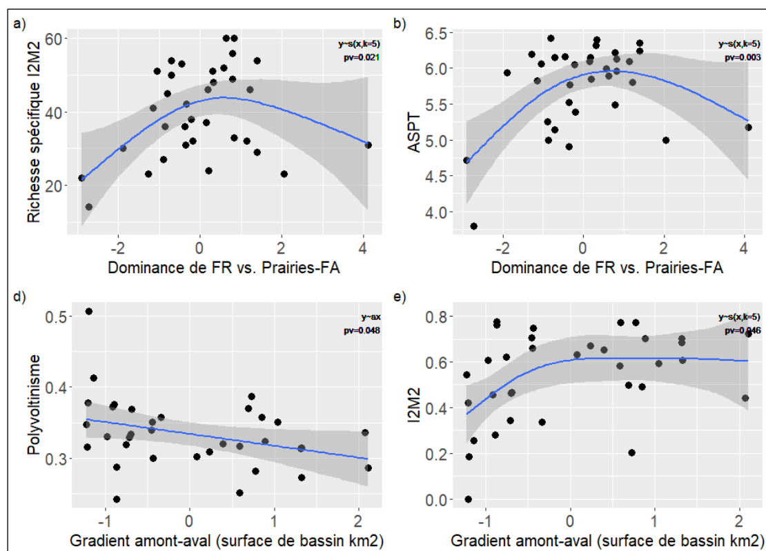
Figure 5 : Principales relations entre la qualité écologique du milieu aquatique, sur la base de métriques de l'I2M2, et les caractéristiques du paysage, le gradient amont-aval. pv=p-value associée à un test de significativité univarié paramétrique ou non paramétrique selon la nature de la relation.
