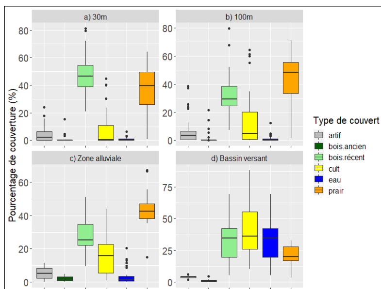
Figure 3 : Distribution des données de pourcentages de couverture par les différents éléments du paysage à travers les quatre échelles d'analyse : a) buffer de 30m, b) buffer de 100m, c) zone alluviale amont de la station et d) bassin versant amont de la station.
