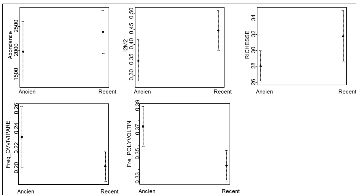
Figure 3 : Moyennes et erreurs standards de quelques métriques de l'I2M2 dans les huit stations selon l'ancienneté de la ripisylve.
