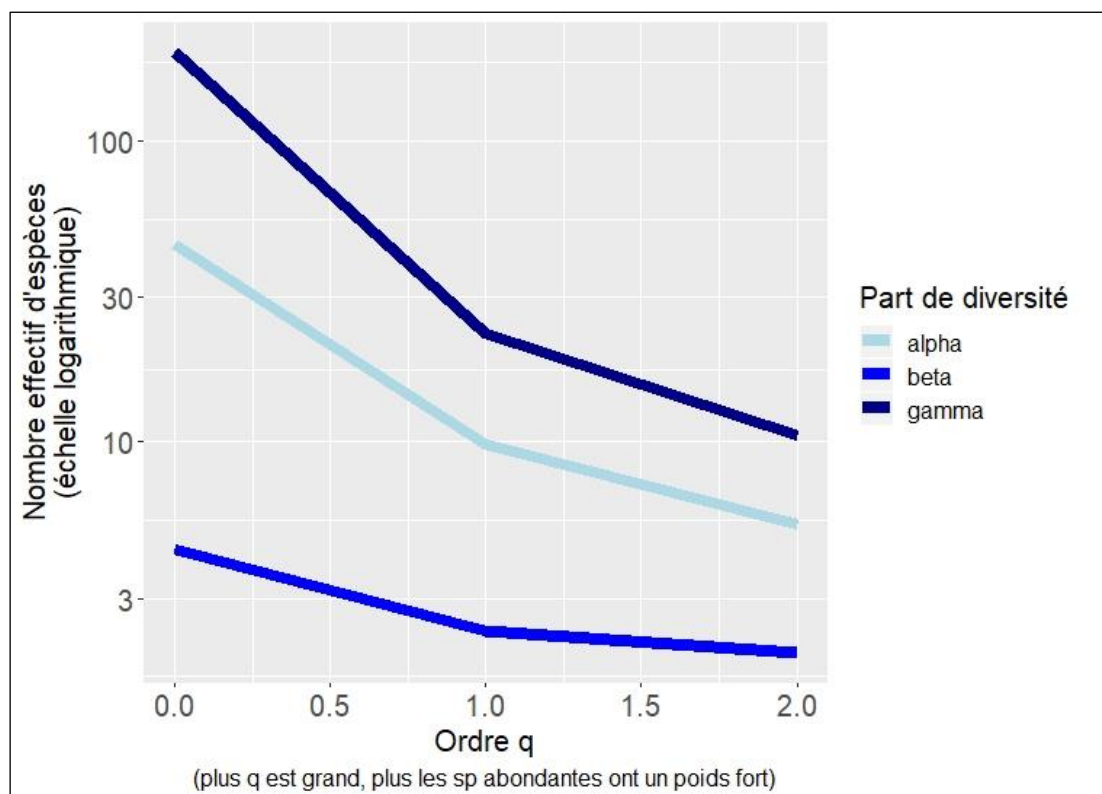
Figure S5.2 : Valeurs de diversités alpha, beta et gamma sur l'ensemble de la zone d'étude exprimées en nombre effectif d'espèces selon l'ordre q. Plus q est grand, plus les espèces communes pèsent dans le calcul de diversité. A contrario, quand q=0 , les espèces faiblement abondantes ont le même poids que les autres dans le calcul (calcul sur la base de la richesse spécifique).
