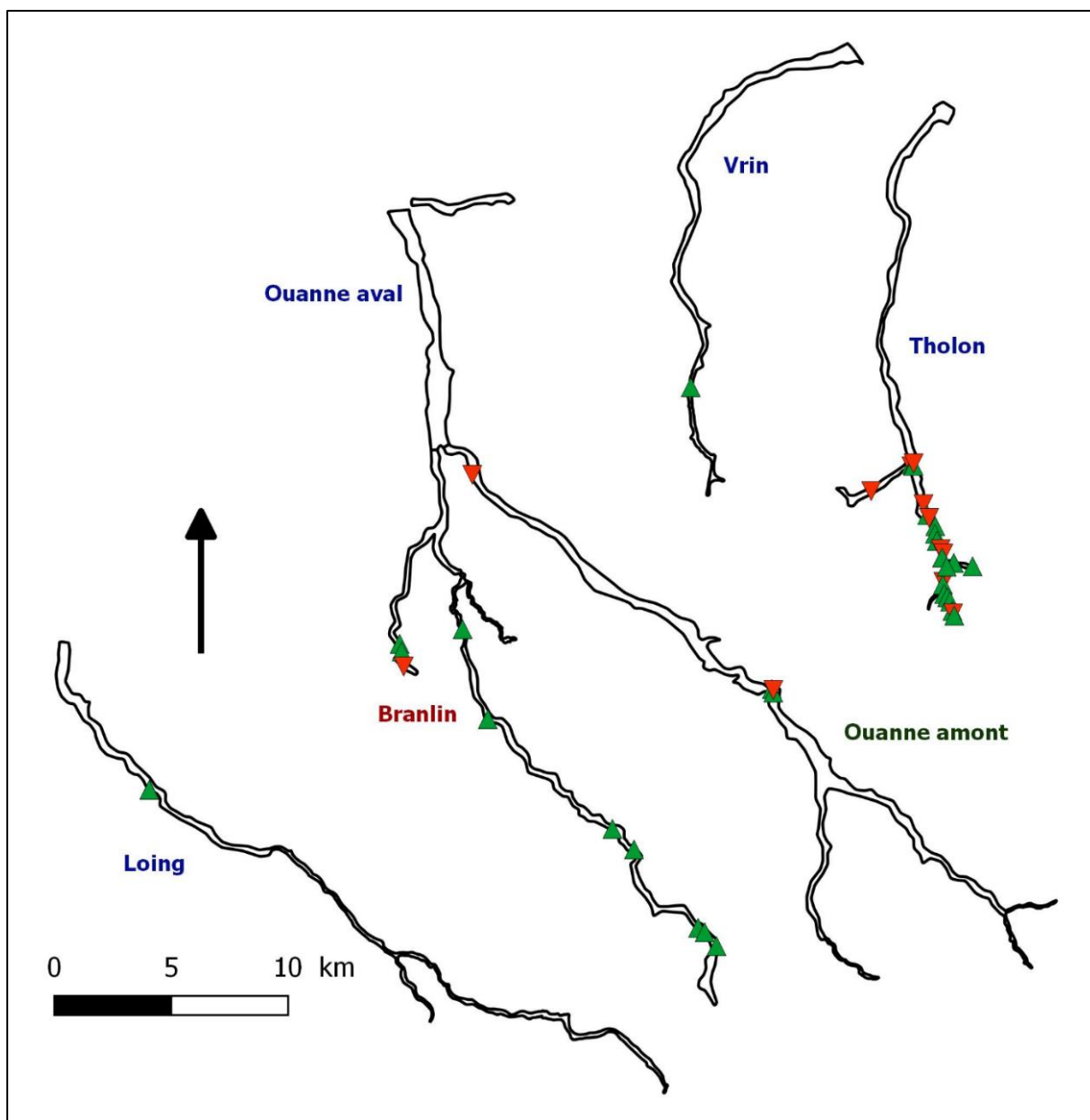
Figure 4 : Carte de répartition des ripisylves anciennes suivant les vallées cartographiées. (Triangles : verts pour bon état de conservation, rouge pour mauvais état).
