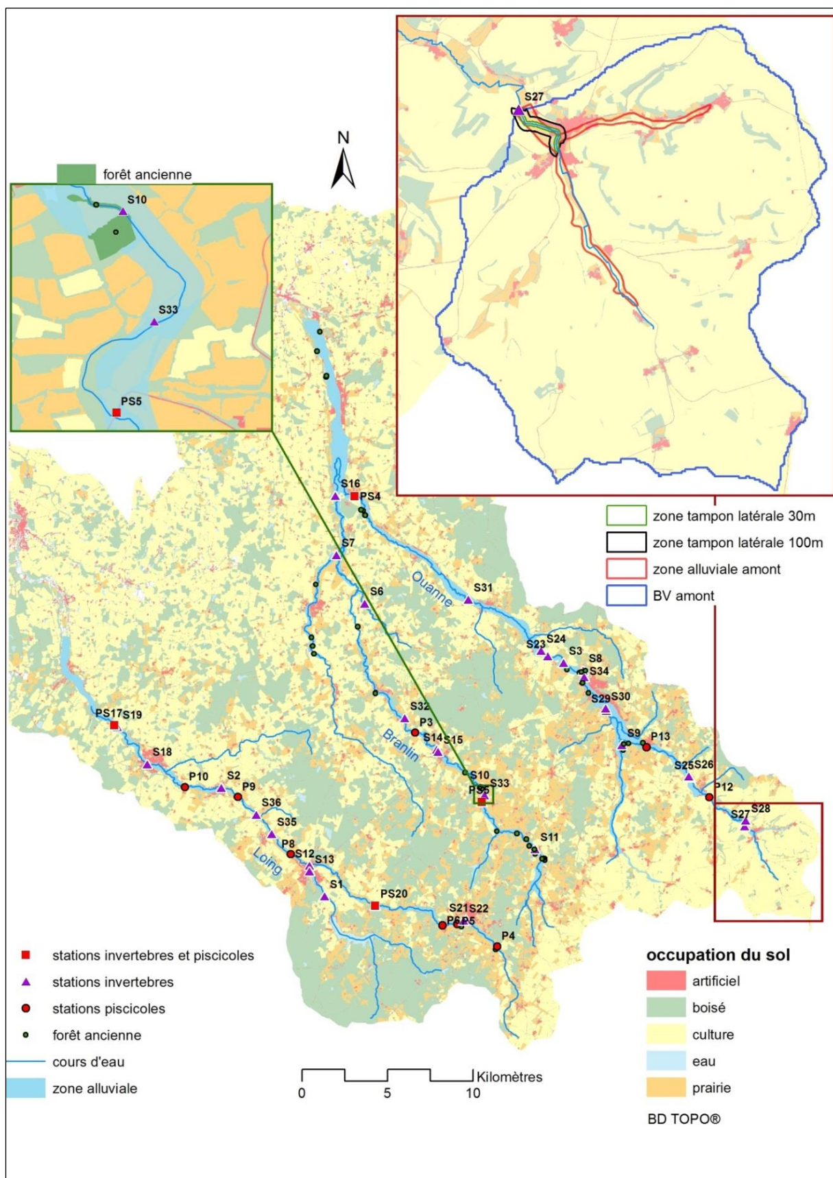
Figure 1 : Répartition spatiale des données utilisées sur les trois cours d'eau étudiés.
