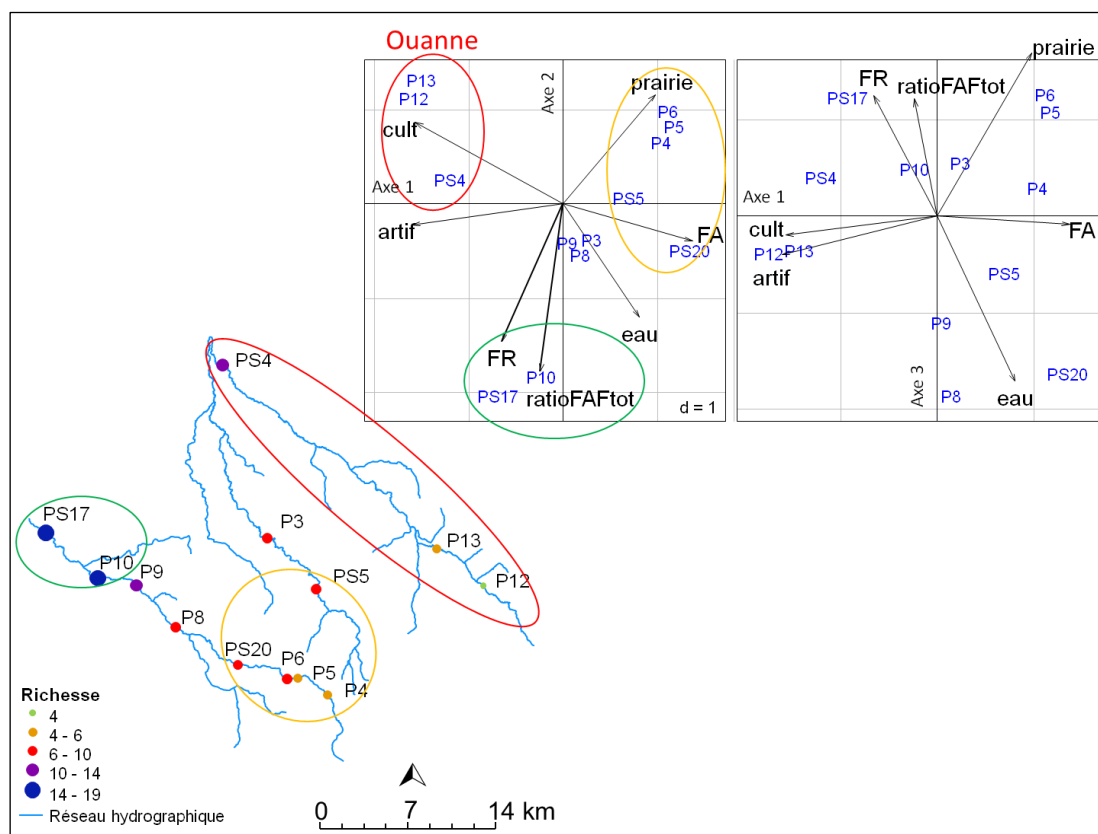
Figure 9 : Richesse spécifique à chaque station d'échantillonnage des poissons et analyse en Composantes Principales (ACP) du paysage à l'échelle alluviale.
