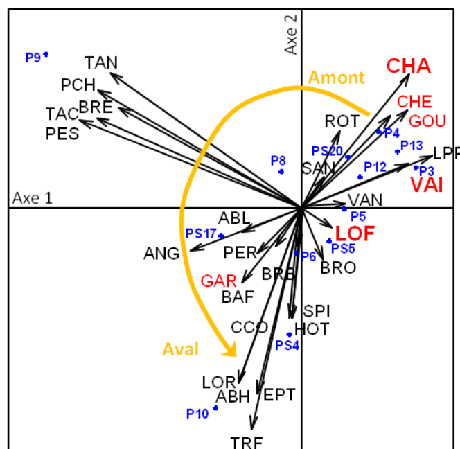
Figure 10 : Analyse du peuplement de poissons par station à l'aide d'une ACP qui donne le même poids aux espèces abondantes ou rares. Les espèces en rouge sont les 6 plus abondantes (cf. Tableau 2), la flèche orange indique une tendance d'évolution des stations de l'amont vers l'aval.
