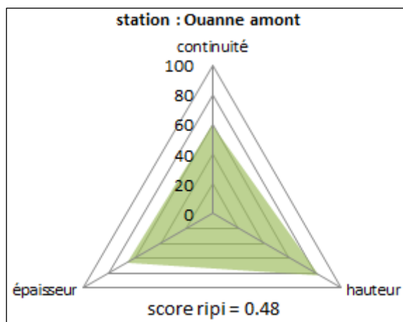
Figure 2 : Exemple de calcul du score ripisylve pour la station Ouanne amont.
