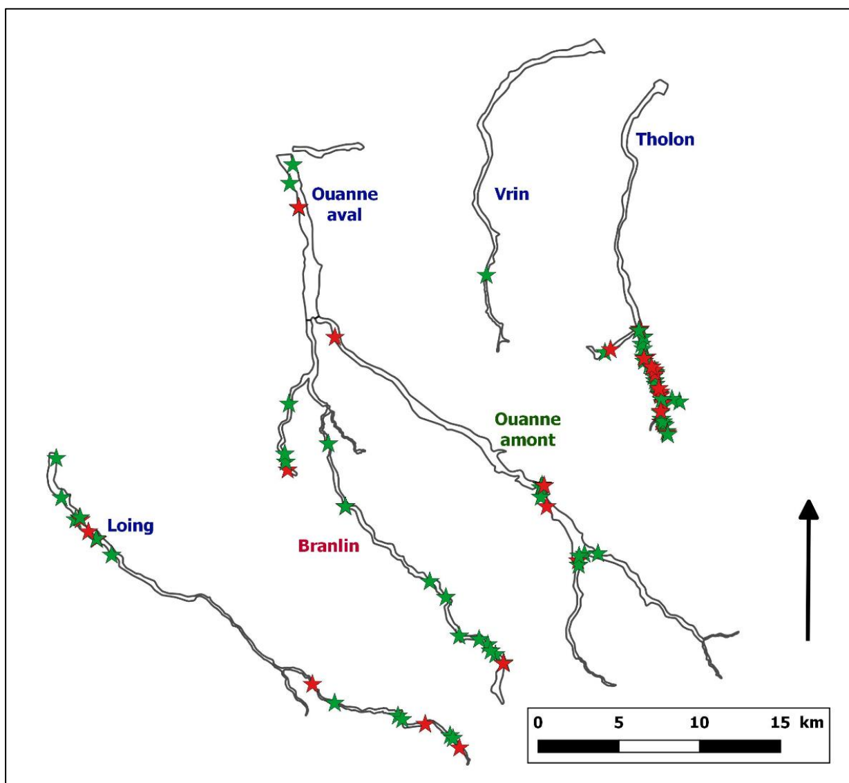
Figure 3 : Carte de répartition des forêts anciennes suivant les vallées cartographiées. (Étoiles : vertes pour bon état de conservation, rouge pour mauvais état).
