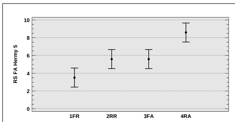
Figure 2 : Progression du nombre d'espèces indicatrices de forêt ancienne (indice Hermey 5) en passant de FR, à RR, à FA et à RR.
