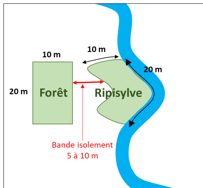
Figure 1 : Agencement des placettes pour la comparaison de la forêt et de la ripisylve. (Source : communication de C. Le Pichon adapté).
